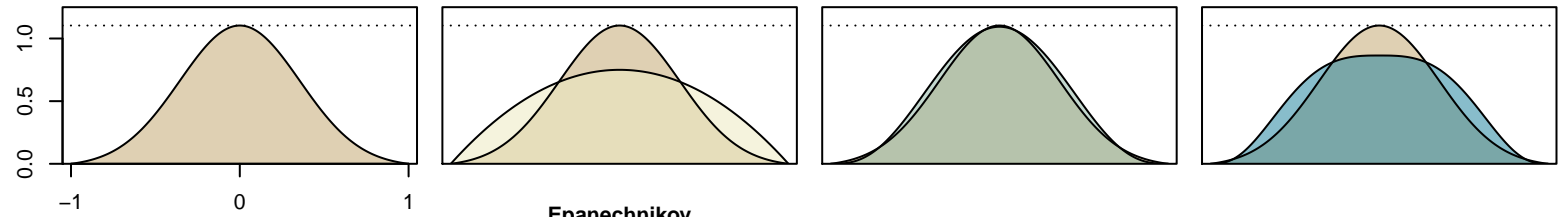
Epanechnikov
